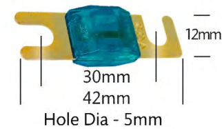
MIDI TYPE FUSE 30A ILU-MIDI-030 40A ILU-MIDI-040 70A ILU-MIDI-070
